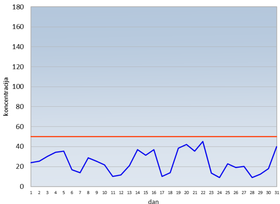
Koncentracija PM u vazduhu mart 2024.
