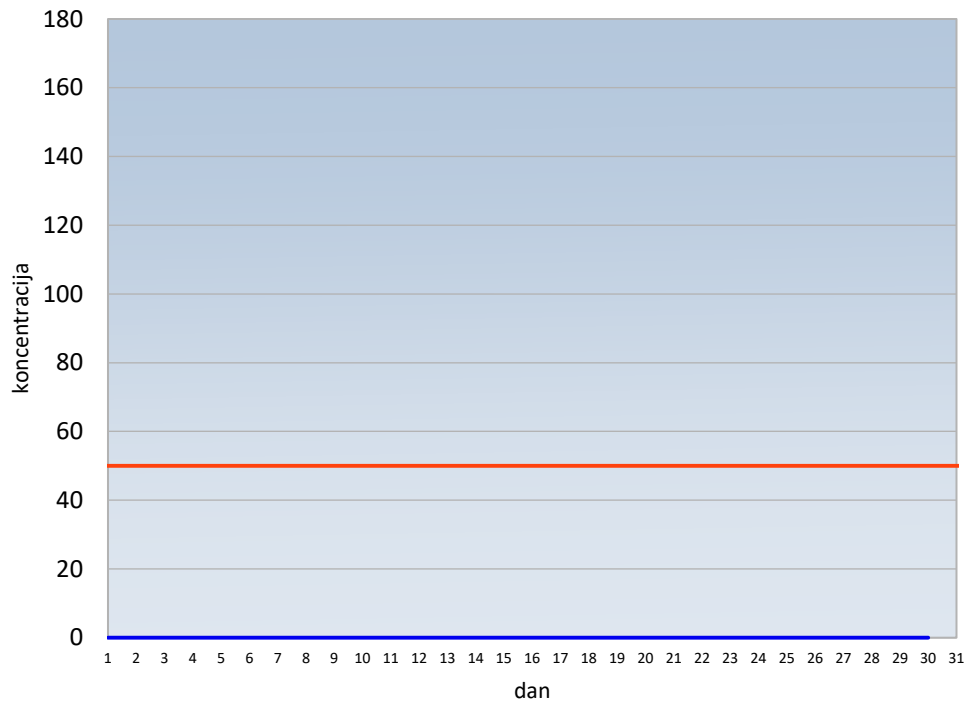
Koncentracija čađi u vazduhu SEPTEMBAR 2024.
